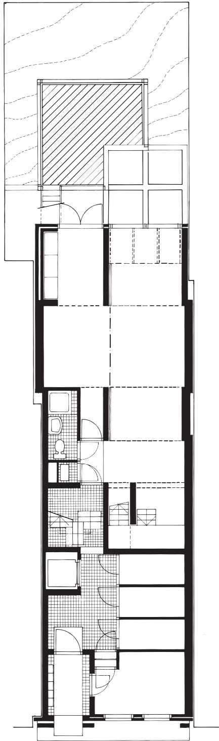
Plattegronden | floorplans
